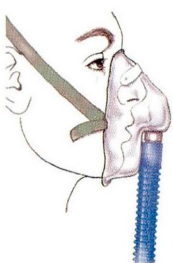
VENTURI MASK
